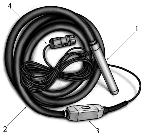
Рис.1 Внешний вид
